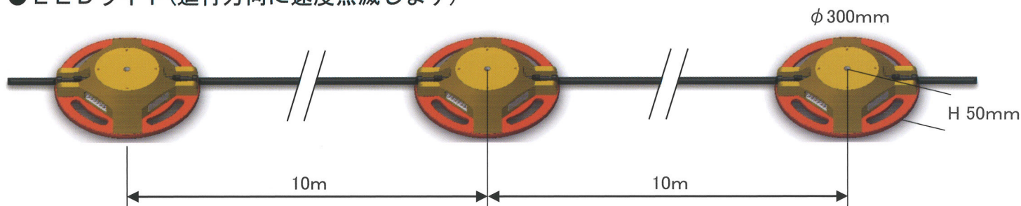
図-1 路面点滅誘導灯の構成
